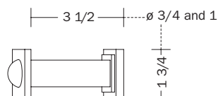
Ligne, holdback
