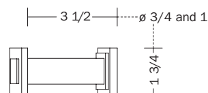
Cône/Carré, holdback
